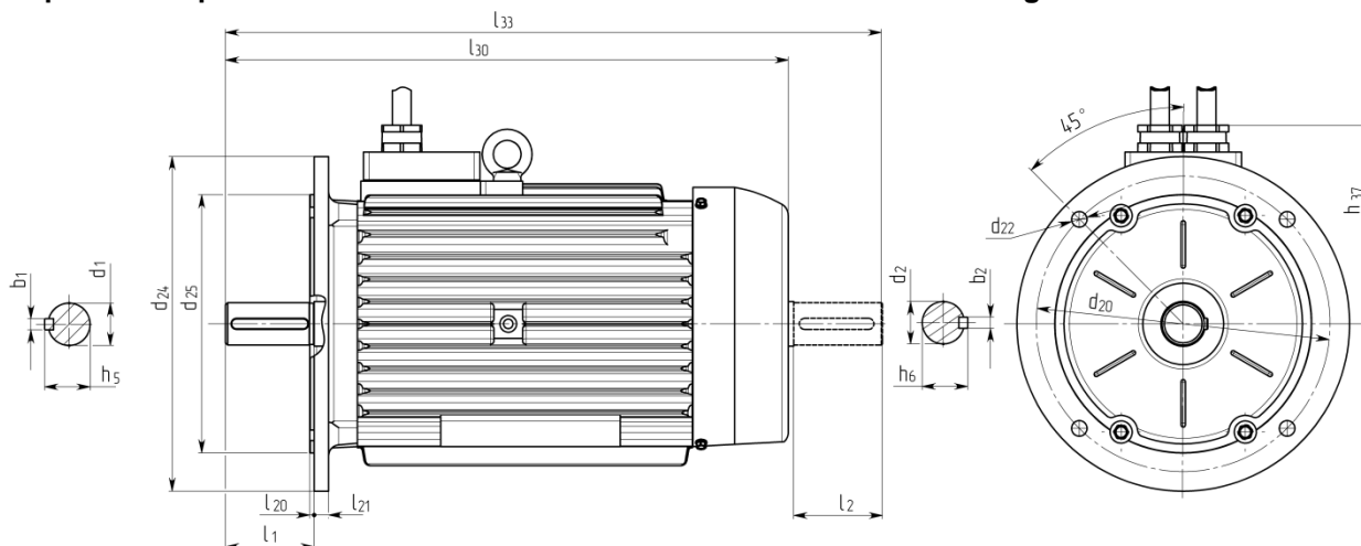
Габаритный чертёж IM 3001 / IM B5.
