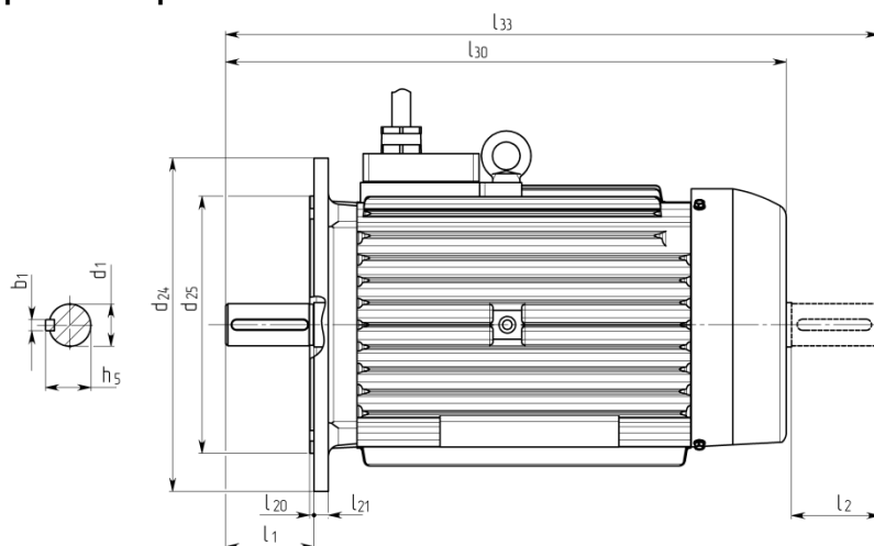
Габаритный чертеж IM 3001 / IM B5.
