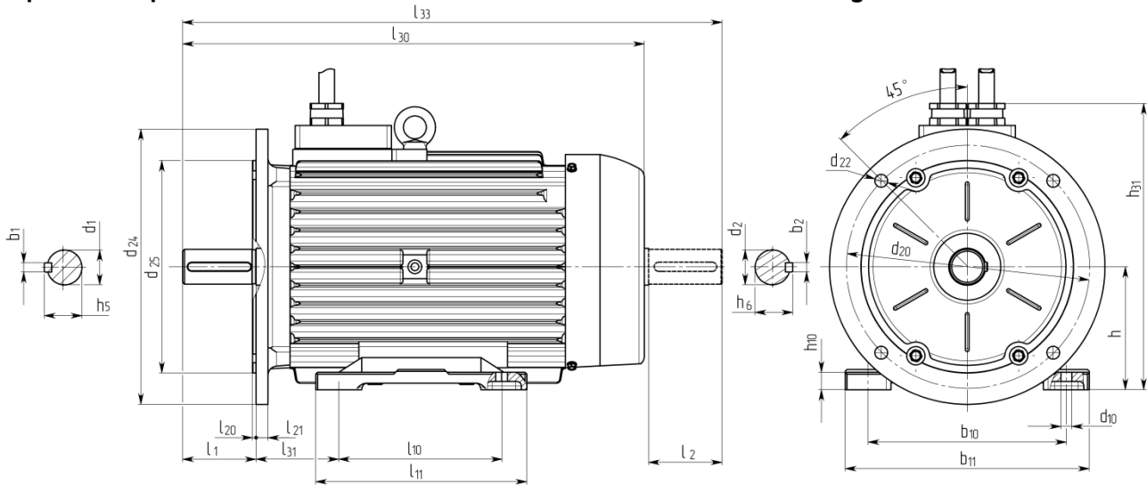
Габаритный чертёж IM 2001 / IM B35.
