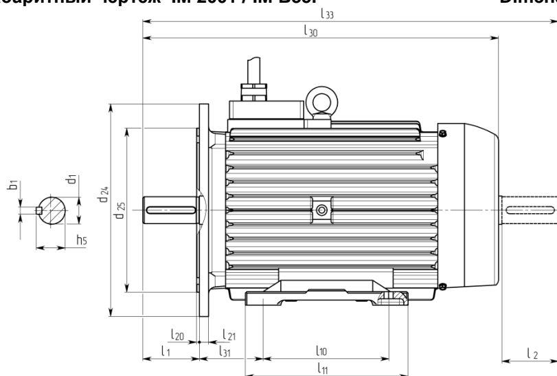
Габаритный чертеж IM 2001 / IM B35.
