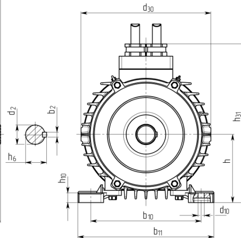
Dimension drawing IM 1001 / IM B3.
