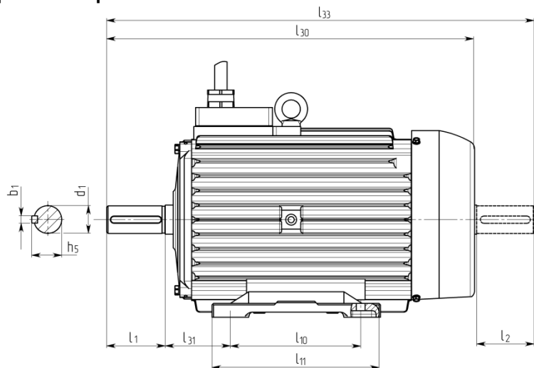
Габаритный чертеж IM 1001 / IM B3.
