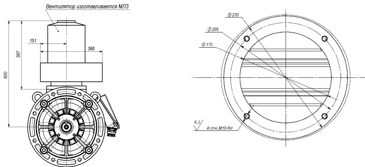
АН200В6/24НЛБФ
